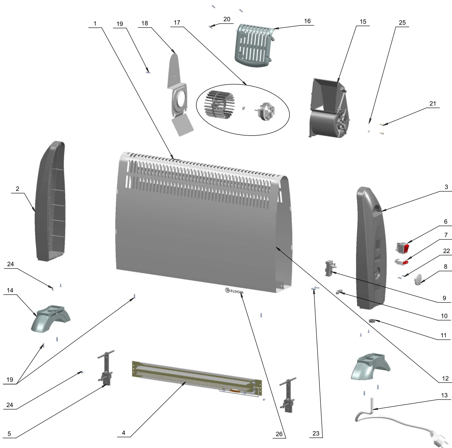
КОНВЕКТОРЕН ОТОПЛИТЕЛ ЗА ПОДОВ МОНТАЖ CF2000/CFV2000 CONVECTOR HEATER FOR FLOOR MOUNTING CF2000/CFV2000
